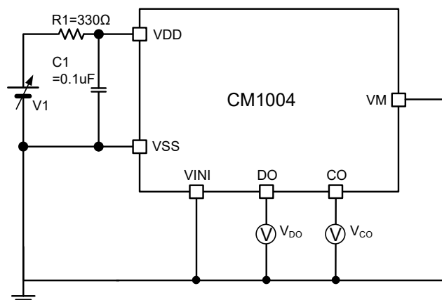
图 8 测试电路 1
