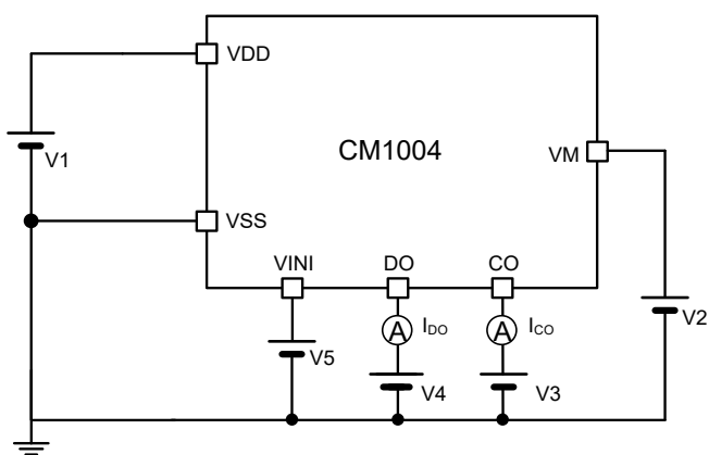
图 11 测试电路 4
