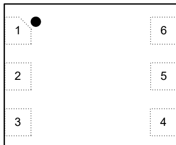
图 2 顶视图
