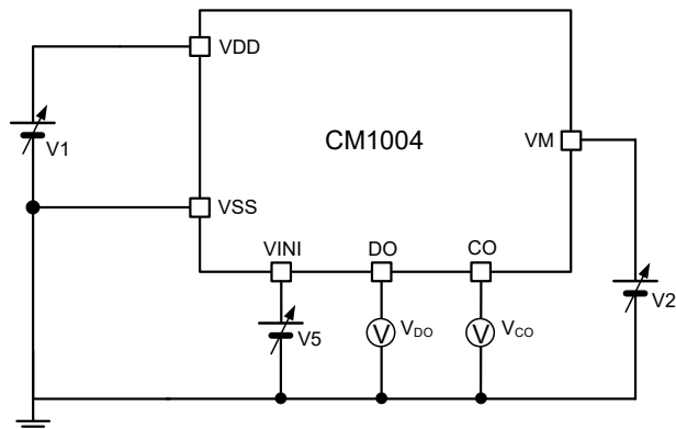
图 9 测试电路 2
