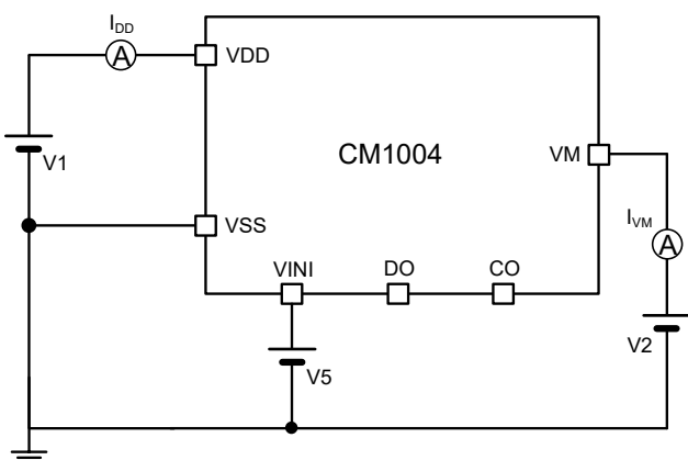
图 10 测试电路 3
