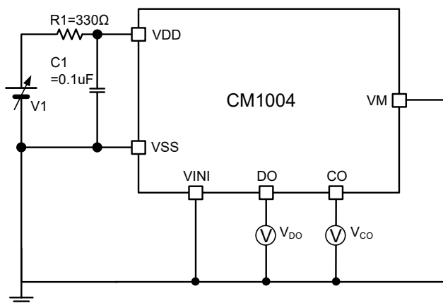
图 8 测试电路 1
