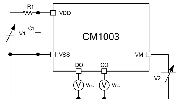
图 8 测试电路 1
