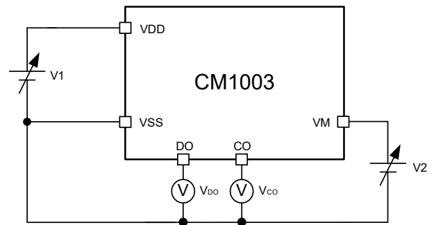
图 9 测试电路 2
