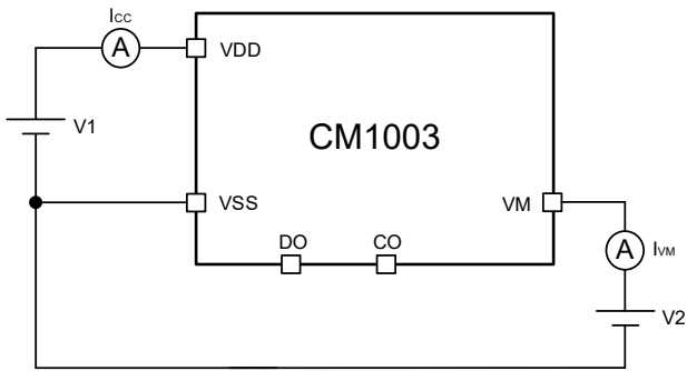
图 10 测试电路 3
