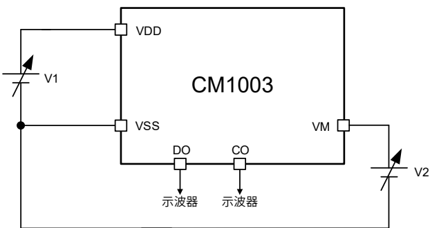
图 12 测试电路 5
