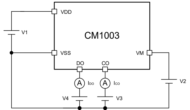
图 11 测试电路 4
