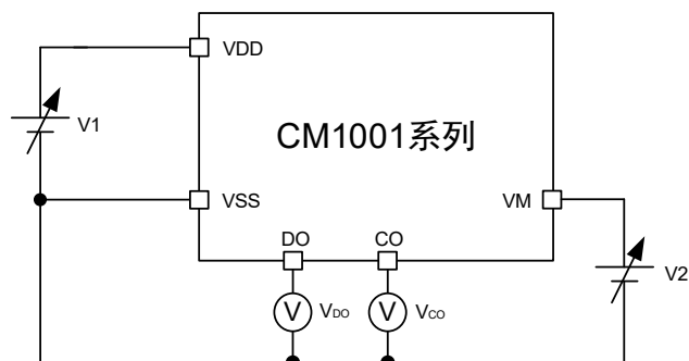
图 8 测试电路 2
